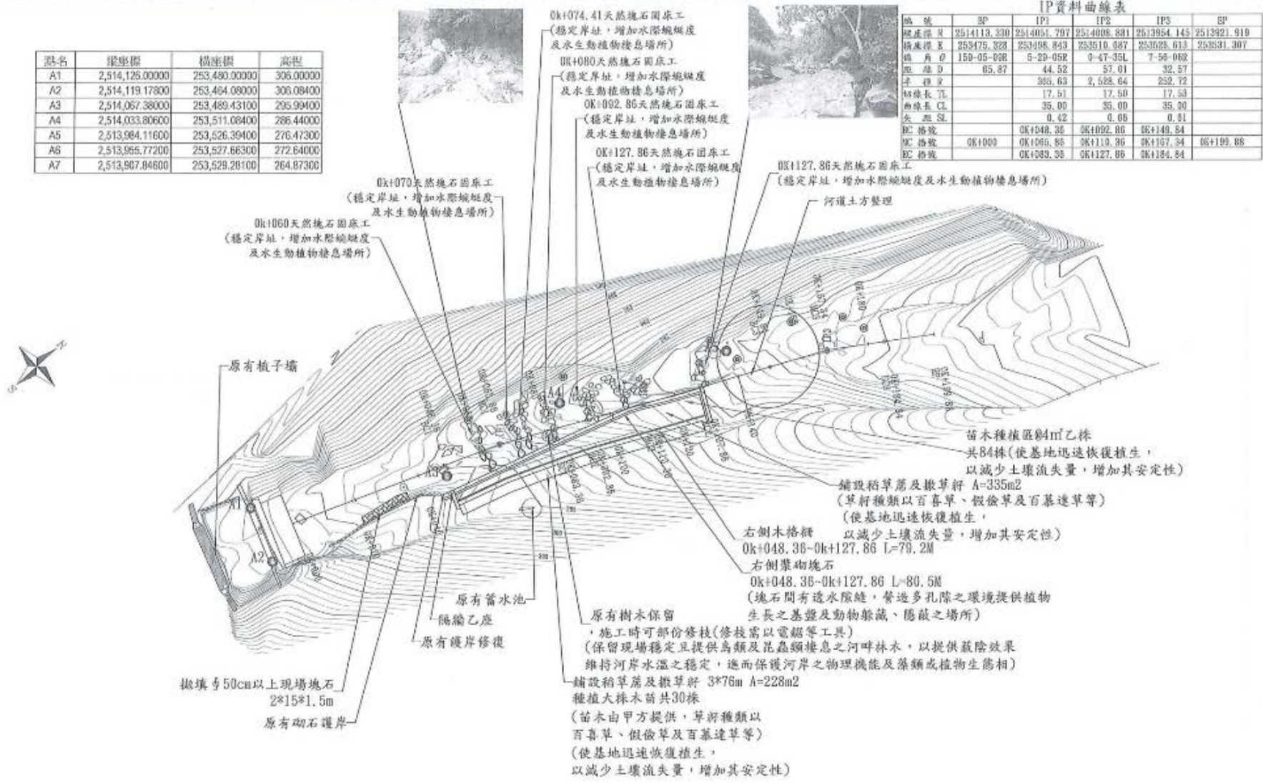
平面圖 S=1/1000
