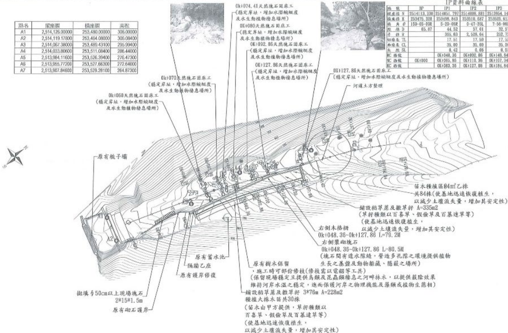
平面圖 S=1/1000
