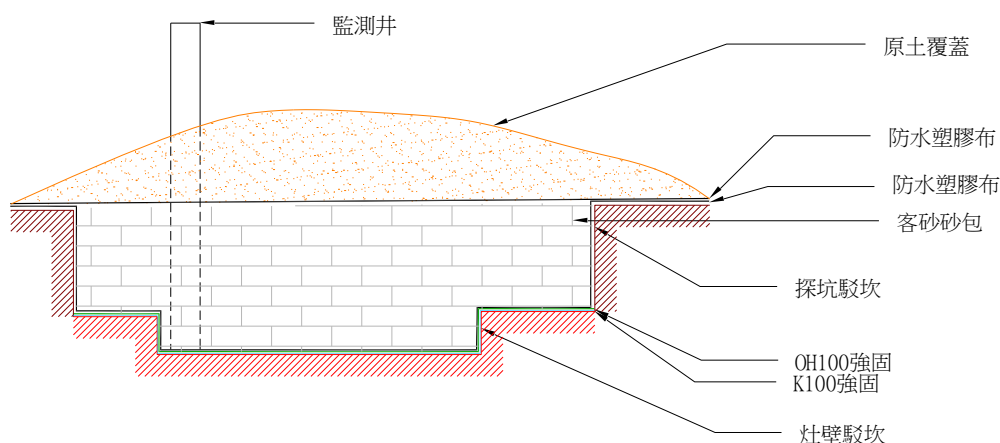
圖 18 道爺南糖廊遺跡臨時強固維護施作工法示意圖
