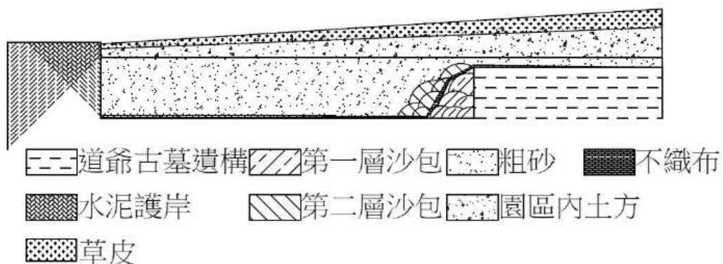
圖 17 道爺古墓回填計畫施工說明書設計剖面圖
